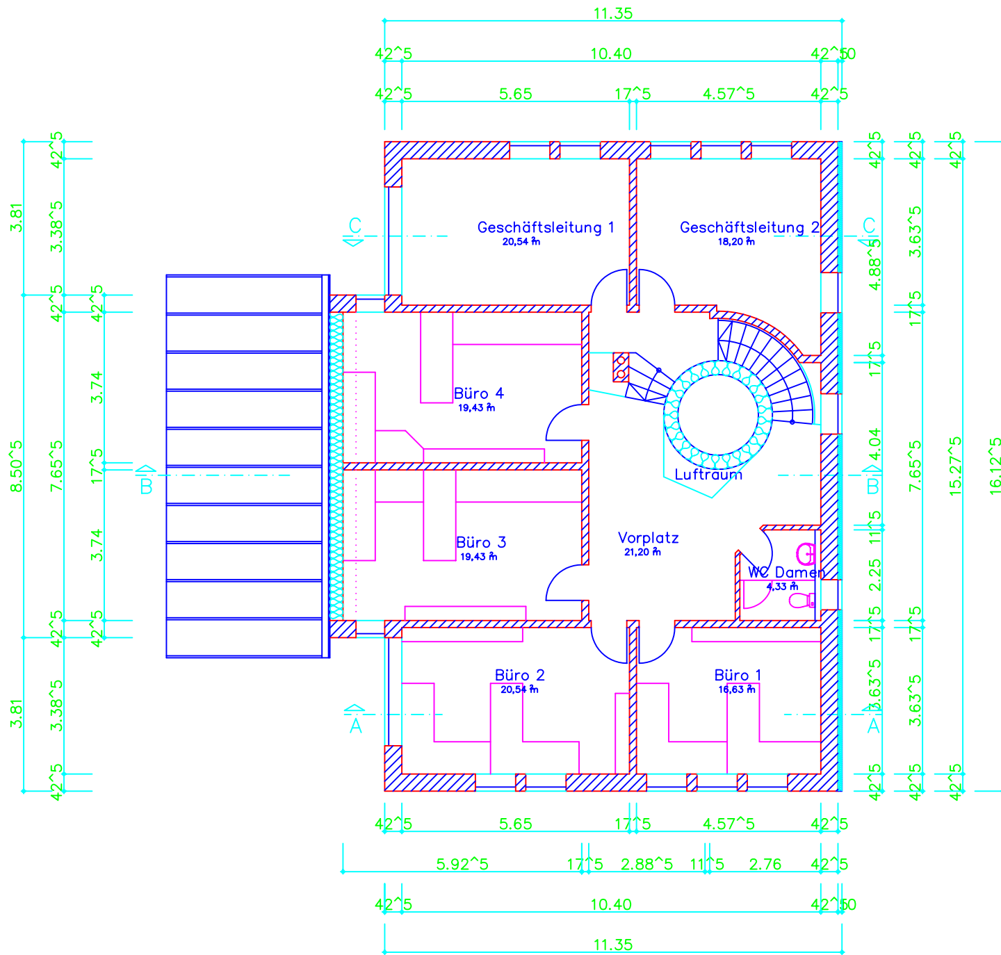
Obergeschoss
